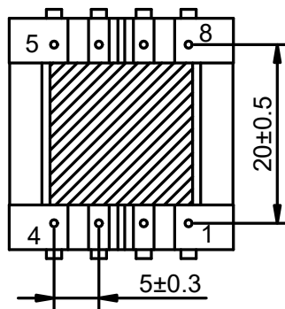
底视图
