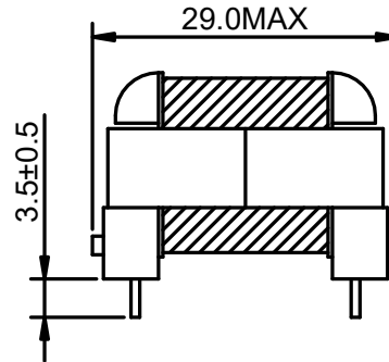
侧视图
