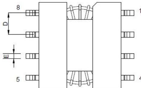
底视图
