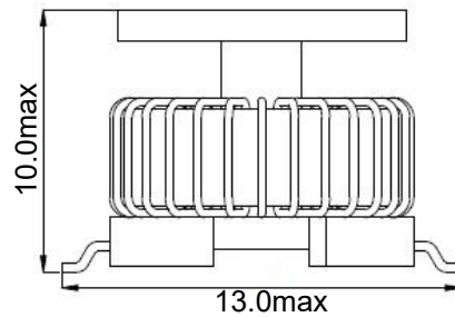
主视图
