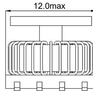
侧视图
